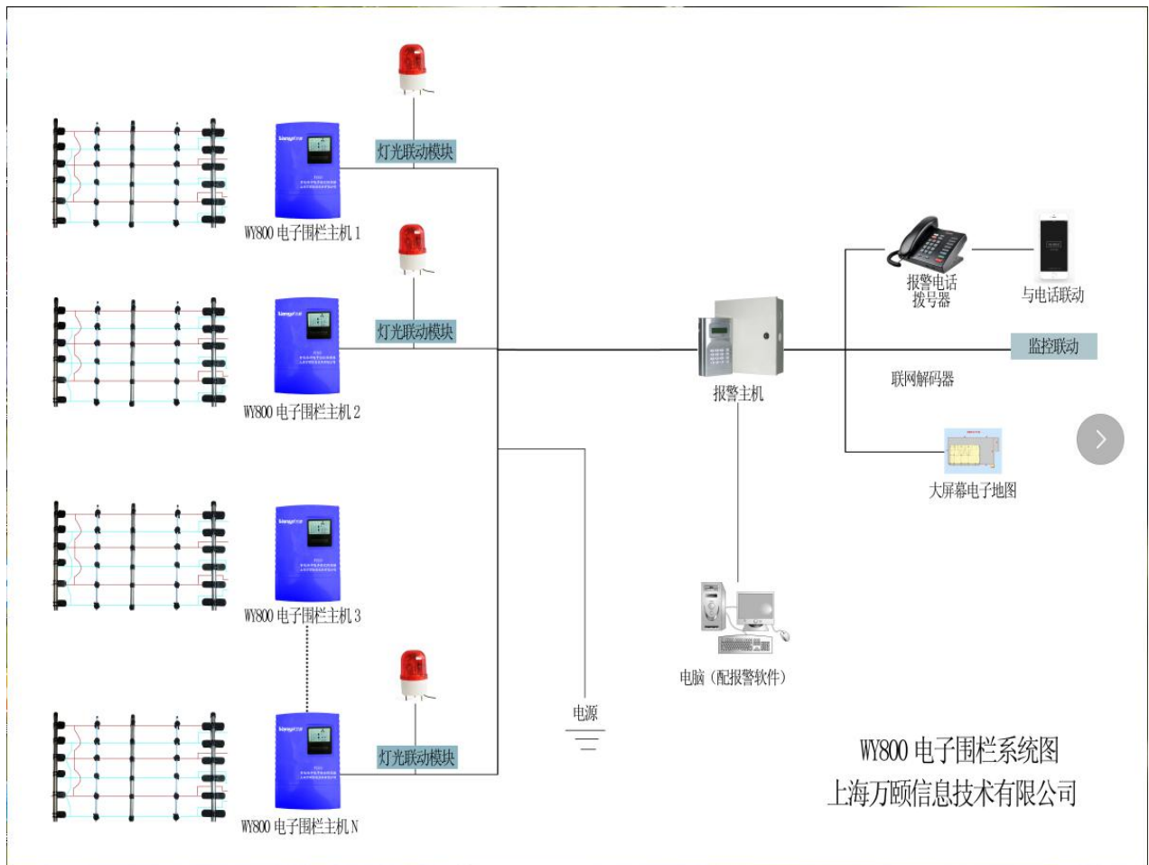
脉冲电子围栏专用控制主机组网系统图
