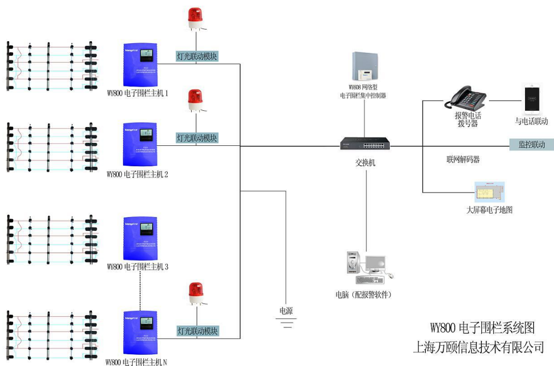
网络型脉冲电子围栏组网系统图
