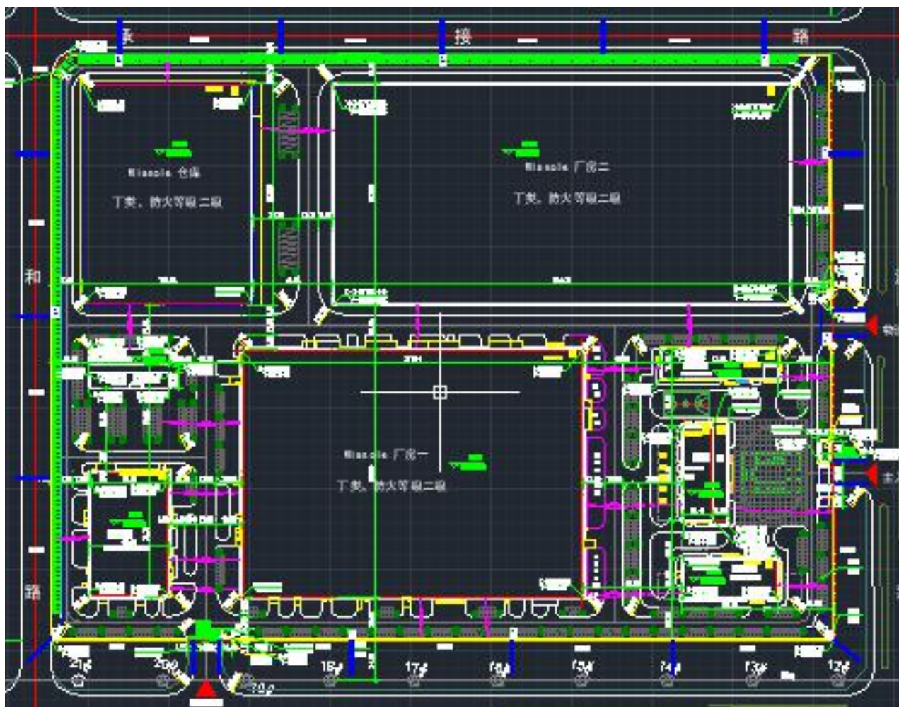
电子围栏防区示意图
